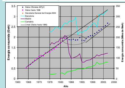
Figura 6. Energía consumida en alumbrado público en puntos (eje izquierdo). Idem en trazo continuo por provincias (eje derecho). La zona plana (marcada en la figura) se explica por el cambio de estadística aplicada en algunas provincias (Madrid, Barcelona, tc).
